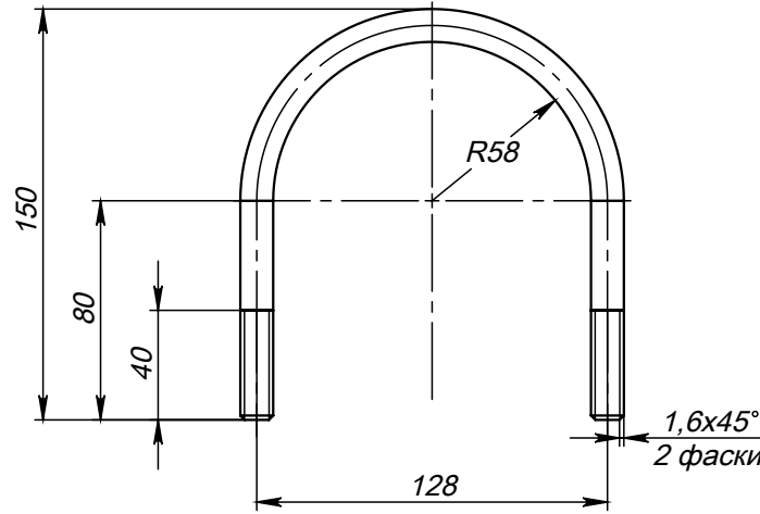
Поз.4 (Хомут)
